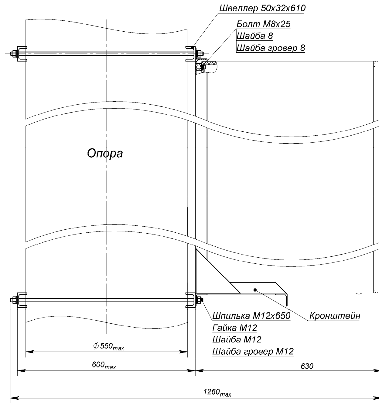
Рис.2 Габаритные и установочные размеры крепления на опору ТШ-9 (ТШ-10)
