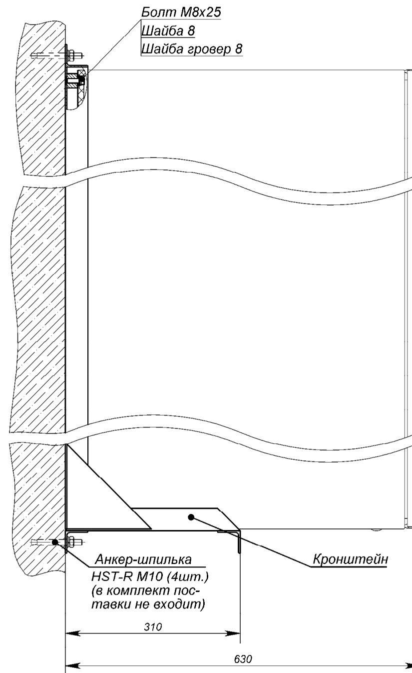
Рис.1 Габаритные и установочные размеры крепления на стену ТШ-9 (ТШ-10)
