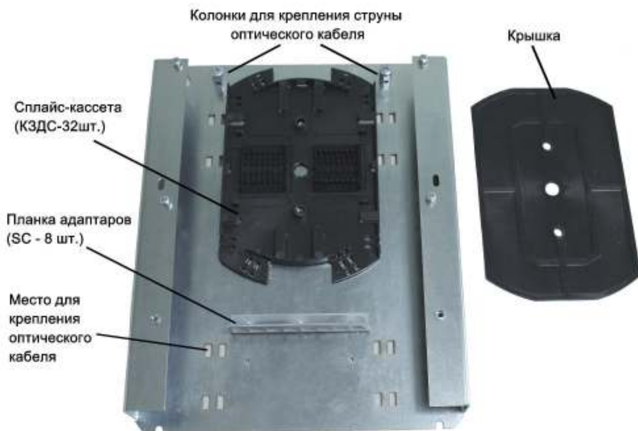
Рисунок 3.3 - Оптический кросс
