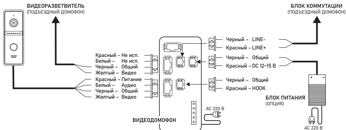
Рис. 24 Схема подключения видеодомофона UNIT 7С к координатному подъездному домофону
