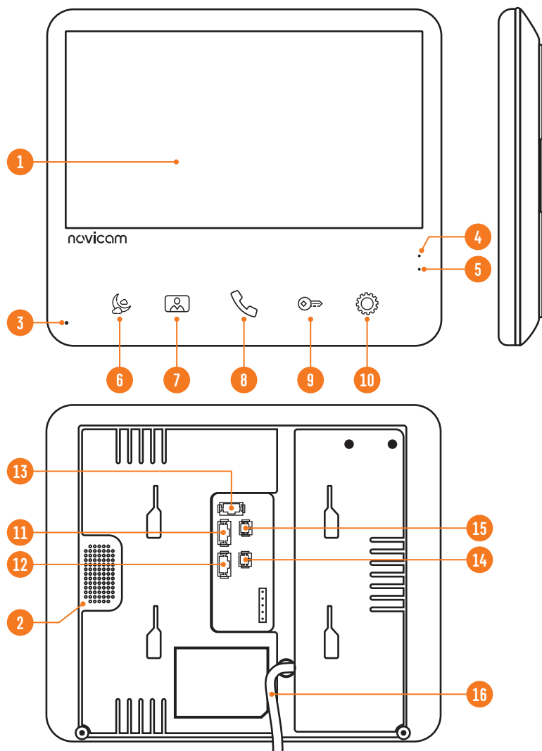
Рис. 5 Видеодомофон UNIT 7
