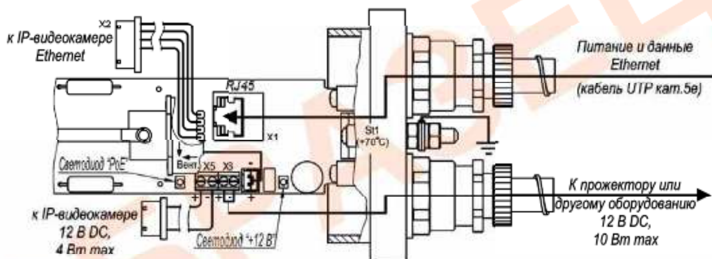
Рисунок 6 – Подключение ТГБ-4М Ex IIC-PoE+
