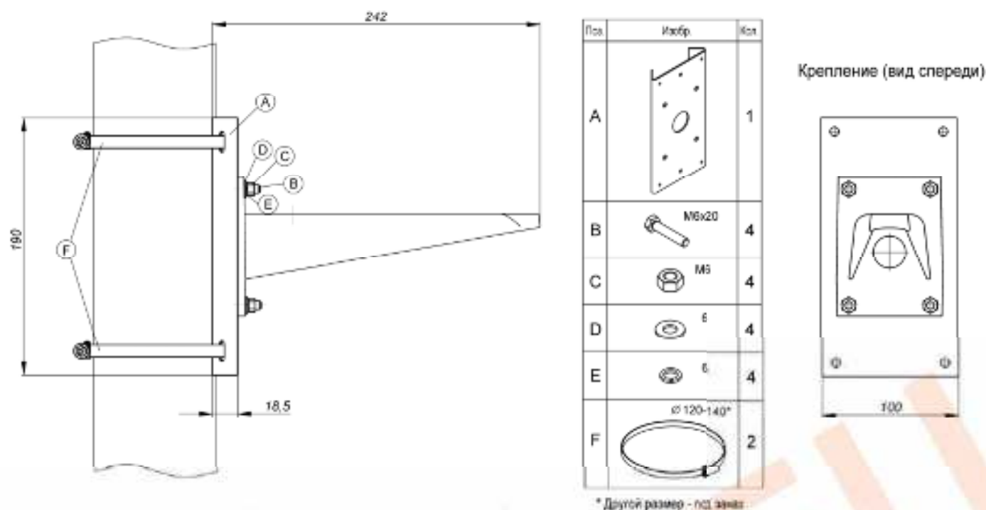
Рисунок 8 – Монтаж кронштейна КС-1 на опору (круглую или квадратную)
