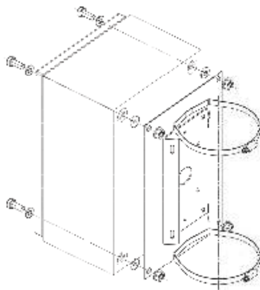
Рис.3 Монтаж кронштейна KS-10 для крепления на квадратные и круглые опоры
