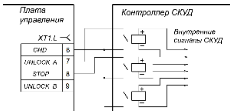
Рисунок 5. Управляющий элемент СКУД – нормально разомкнутый контакт реле
