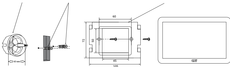
Монтажная коробка
