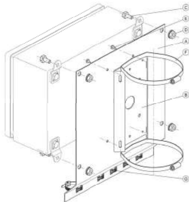
Рис.2 Монтаж кронштейна КС-5 для крепления КМ-7 на квадратные и круглые опоры
