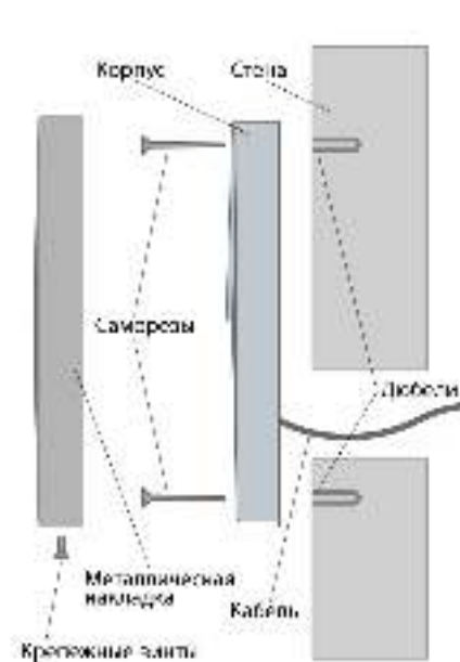
Рисунок 2. Крепление считывателя PNR-P15
