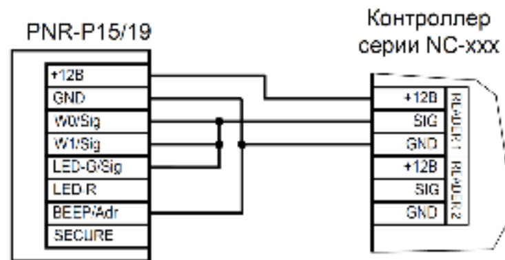
Рисунок 8. Подключение считывателя по интерфейсу Parsec, адрес 0 (наружный)
