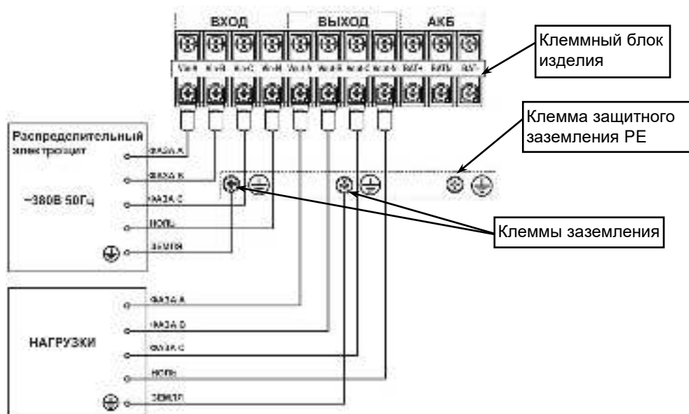
Рисунок 23 — Схема подключения изделия.
