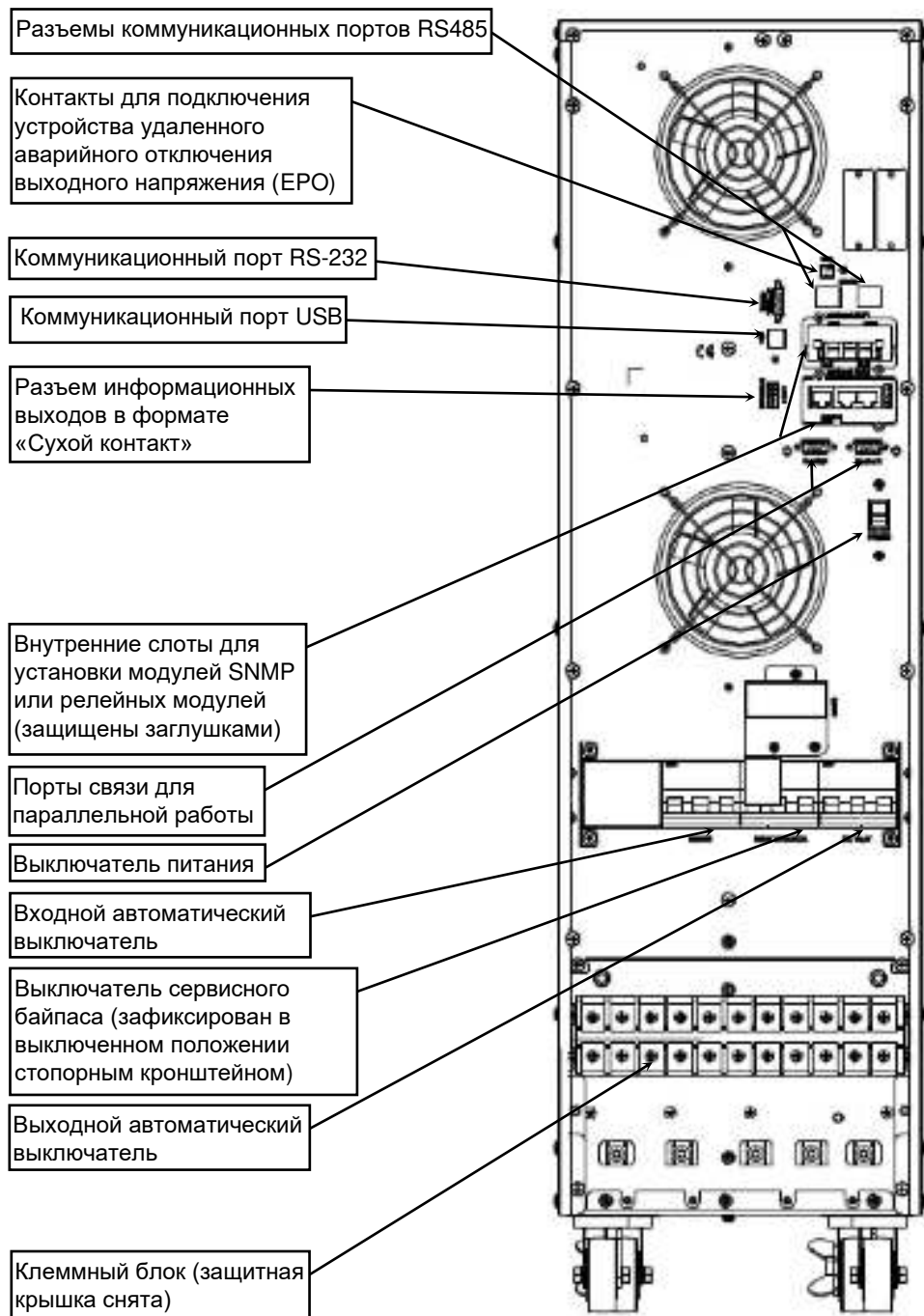
Рисунок 2.2 — Общий вид задней панели изделий SKAT-UPS 15-3/3-ON-2х(20х9) и SKAT-UPS 20-3/3-ON-2х(20х9) со снятой крышкой клеммного блока
