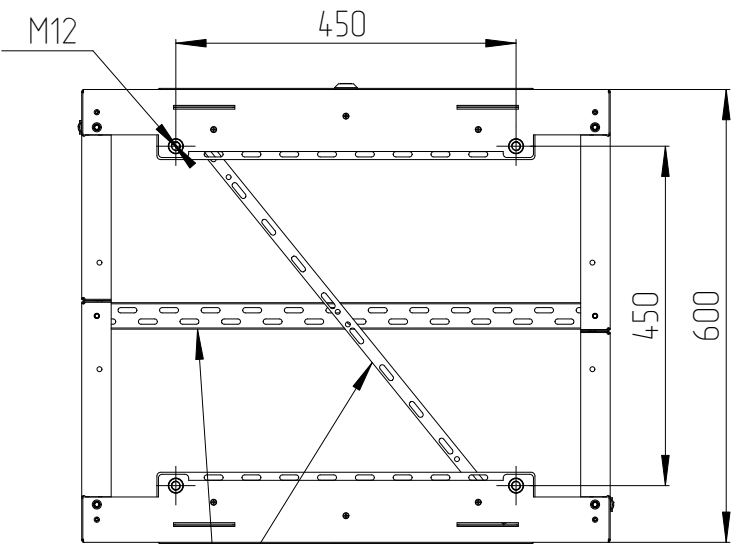
Цоколь ОС-ШТВ-1-300.600
