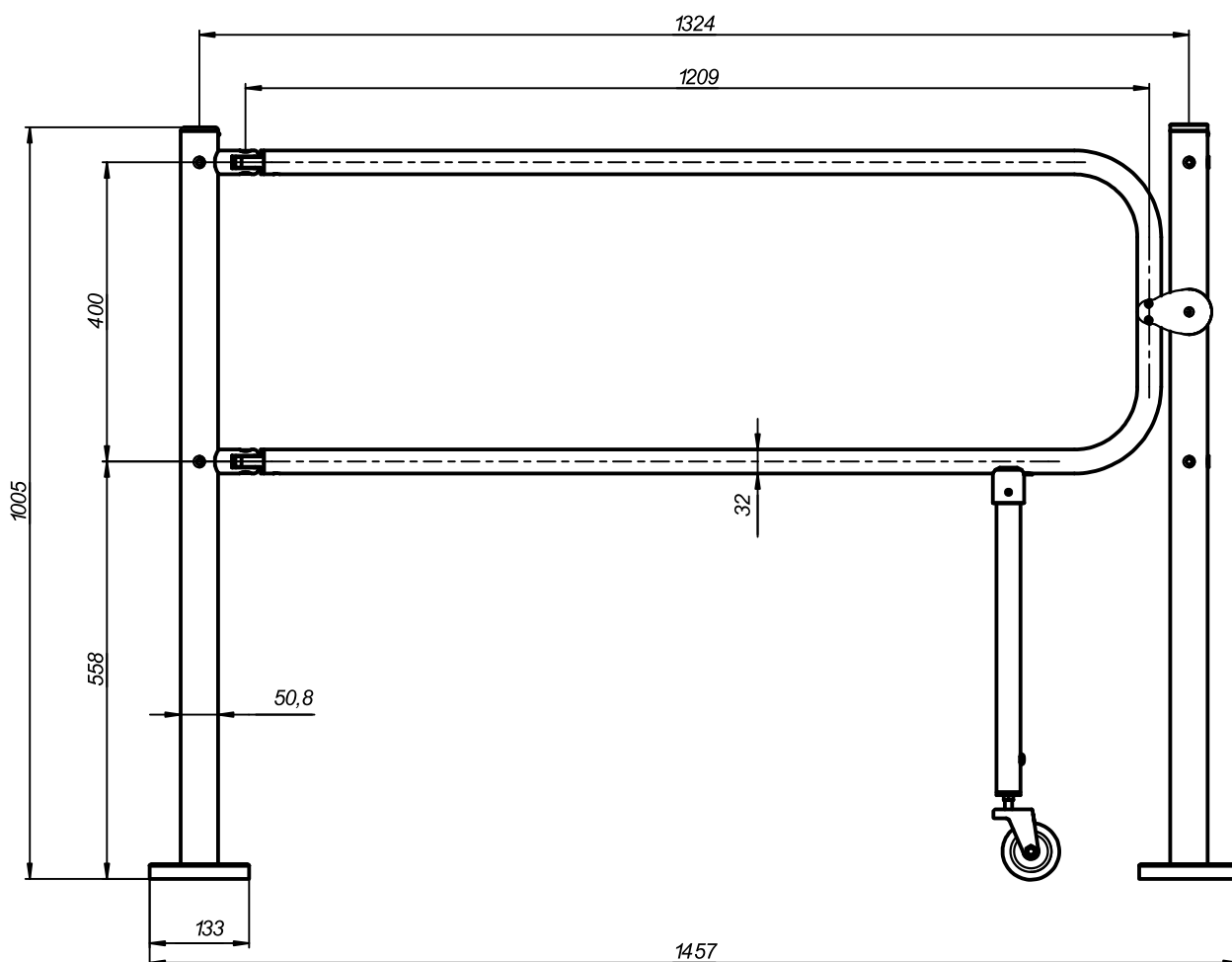
Рисунок 1. Габаритные размеры секции «Антипаника» с электромагнитным замком серии «ХТА-02».
