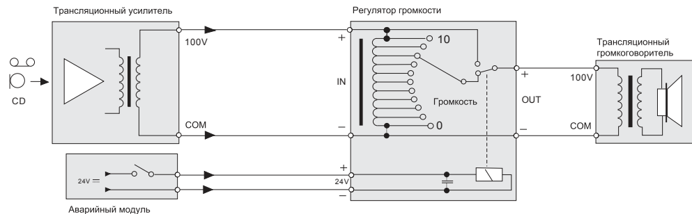
Схема подключения
