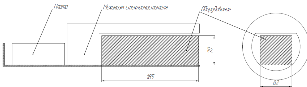
Рисунок А2 – Полезный объем термокожуха для установки видеооборудования – 82x70x190 (габариты видеооборудования, ШxВxГ, мм)
