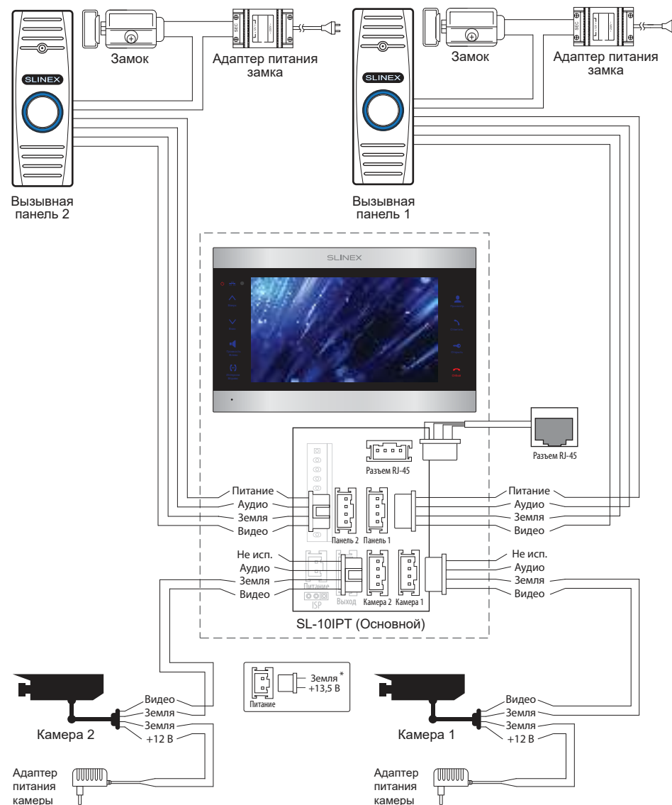
Схема 1. Подключение вызывных панелей и камер к домофону SL-10IPT.
