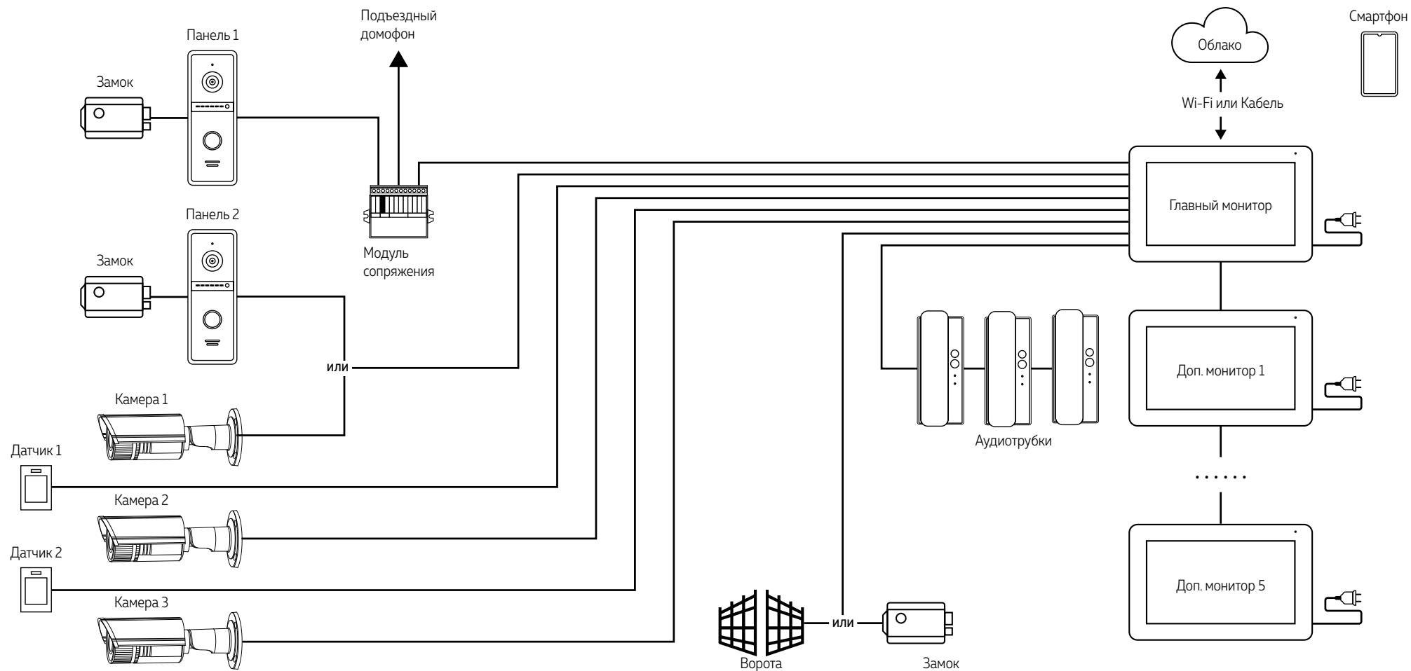
Рис. 8 Структурная схема системы на базе видеодомофонов FREEDOM
