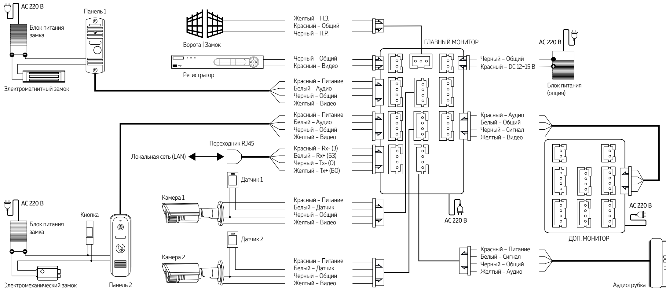
Рис. 9 Схема подключения видеодомофонов FREEDOM
