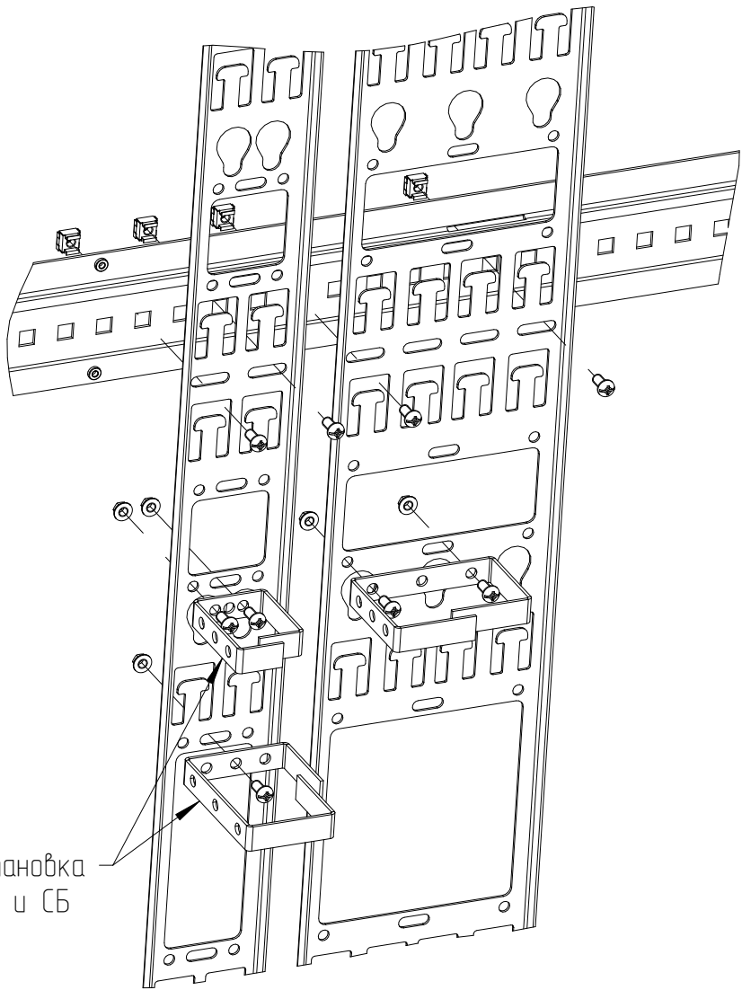
Пример крепления ВКО-М
