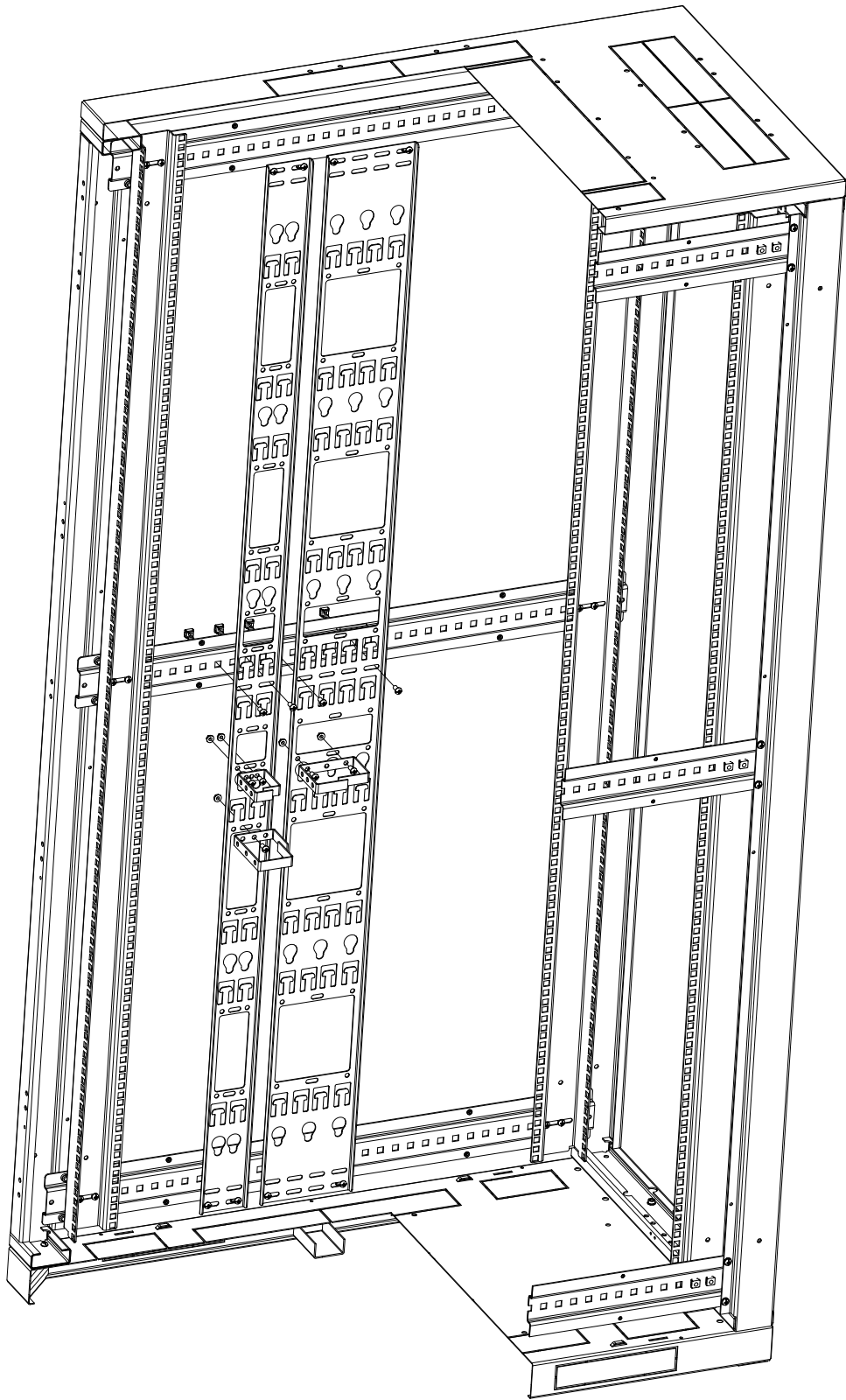
Установка СМ и СБ
