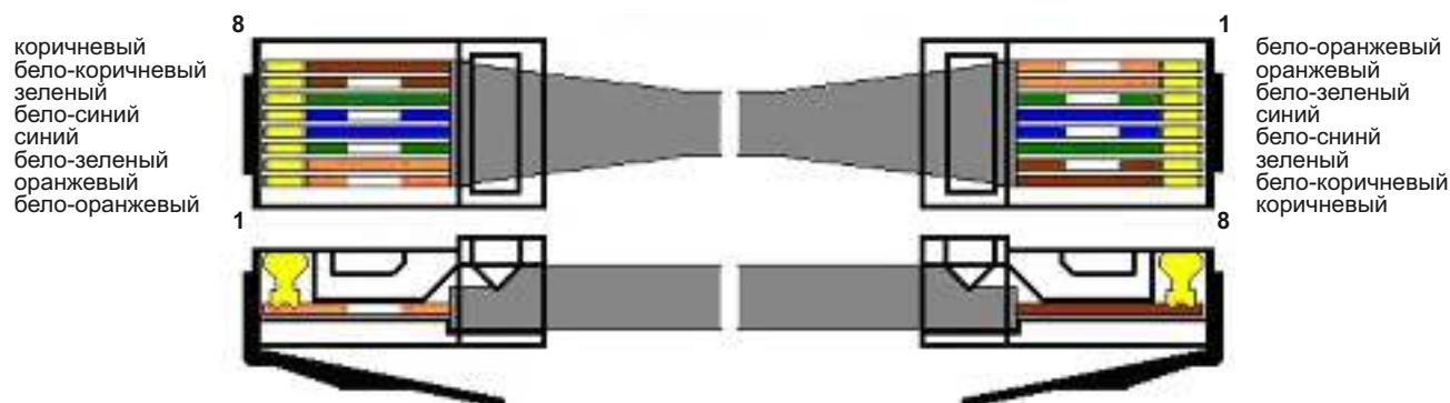
Рисунок 6 - Схема обжимки кабеля UTP Cat5 - прямой патч-корд
