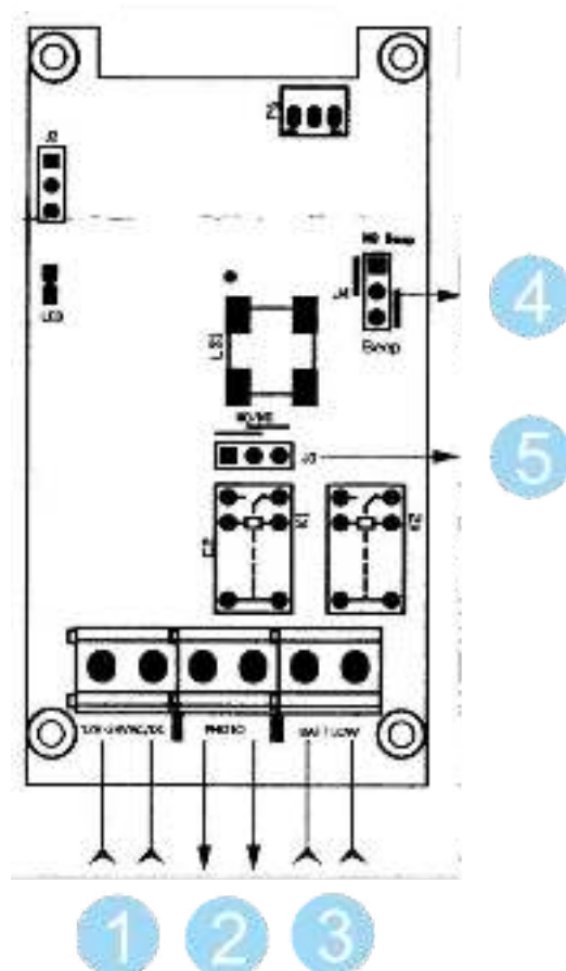
Рисунок 6.7.1.6 Устройство платы приемника
