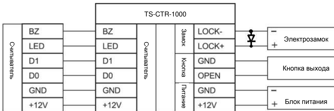
Рисунок 2: Схема подключения
