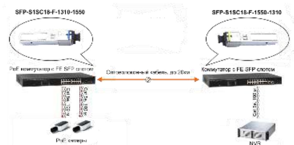
Рис.4 Типовая схема подключения SFP модулей SFP-S1SC18-F-1310-1550, SFP-S15C18-F-1550-1310
