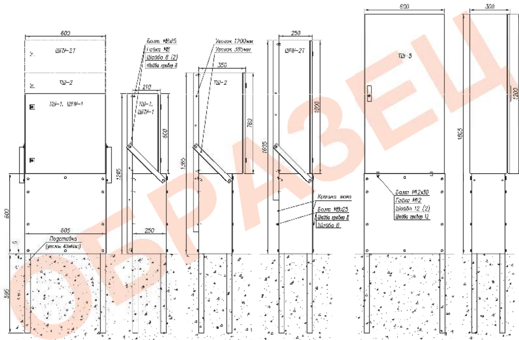
Рис.1 Габаритные и установочные размеры основания мобильного ОНШ-2.
