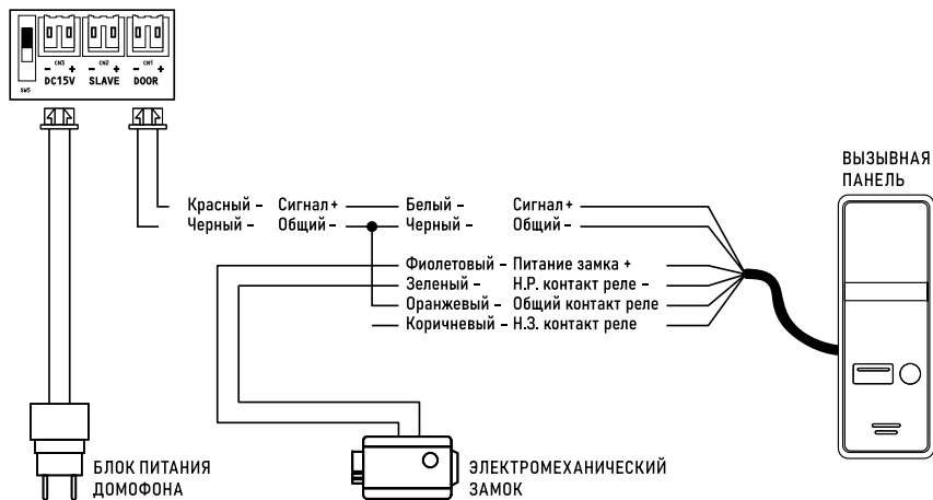
Рис.1 Схема подключения аудиодомофона к электромеханическому замку
