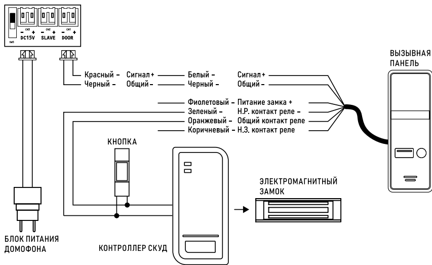
Рис.2 Схема подключения аудиодомофона к СКУД и электромагнитному замку
