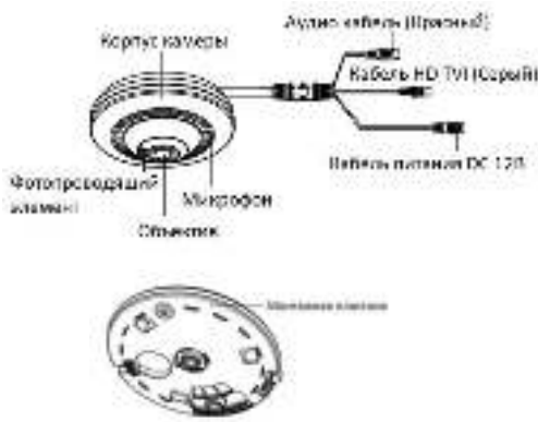
Рисунок 1-1 Внешний вид камеры
