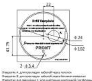
Рисунок 2-1 Шаблон крепления
