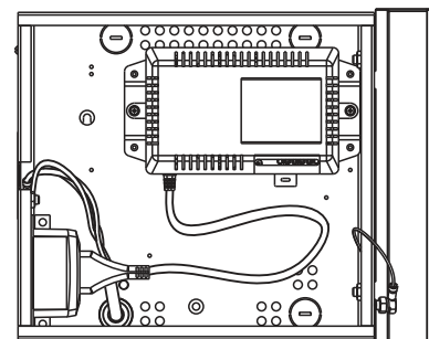
Рисунок 5 - Расположение блока питания VIZIT в боксе
