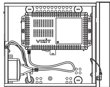
Рисунок 4 - Расположение блока управления VIZIT в боксе
