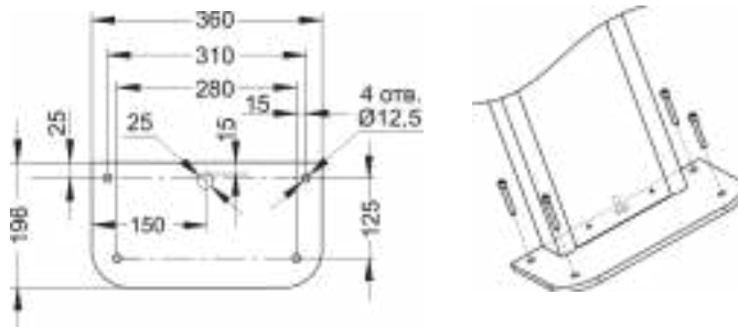
Рисунок 5. Установка турникета на основание
