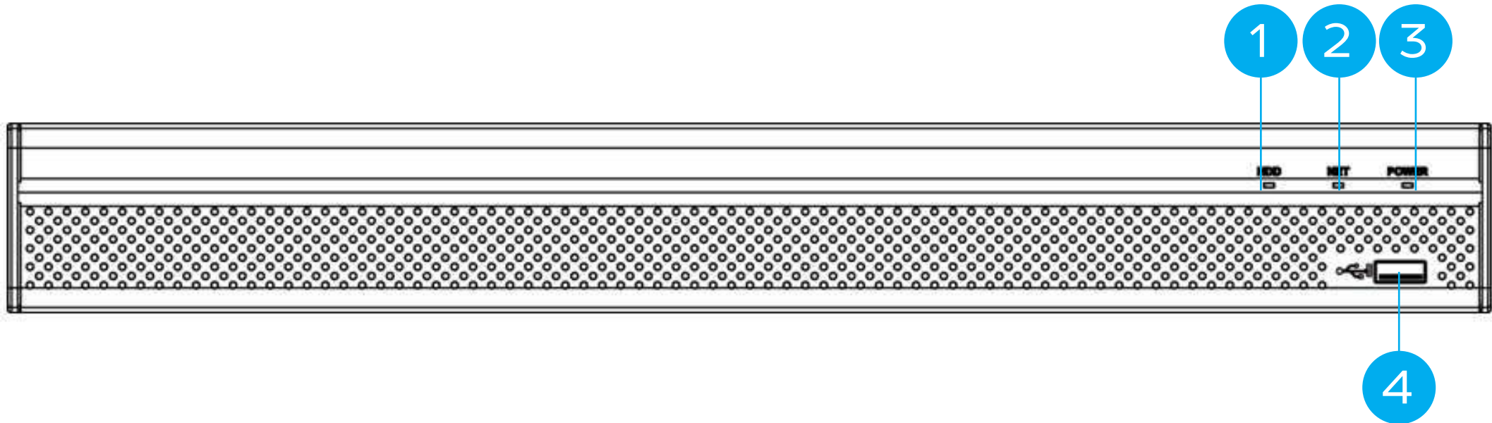
Передняя панель
