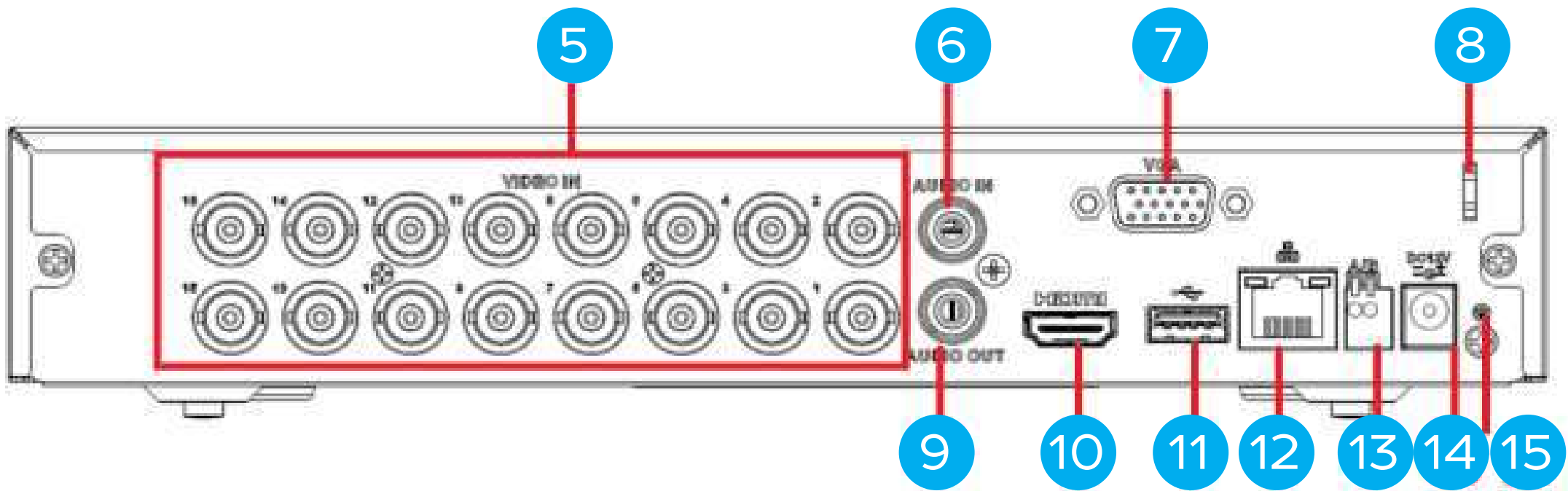
Задняя панель
