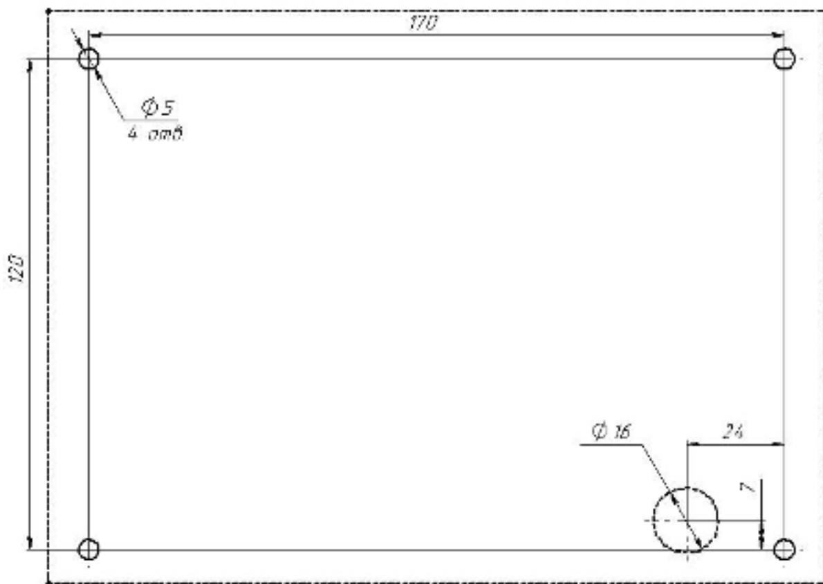
Рис. 2 Разметка отверстий для установки контроллера (Пунктиром показаны габариты корпуса и примерное место для отверстия под кабели.)
