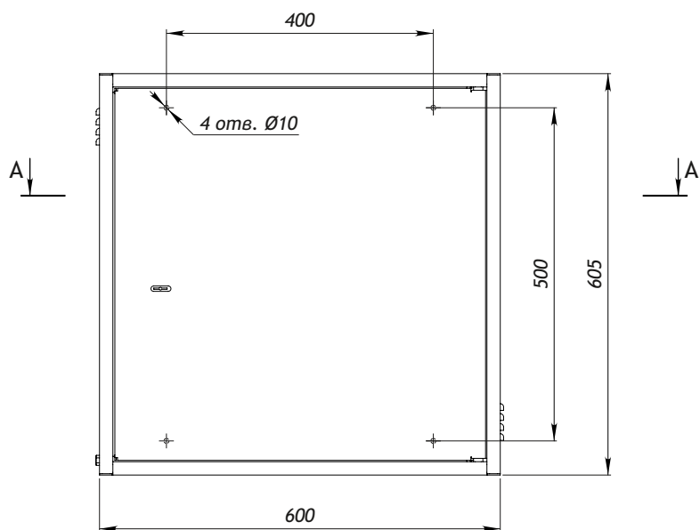
Сечение А-А
