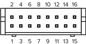
Рис. 12. Расположение контактов шлейфового разъема
