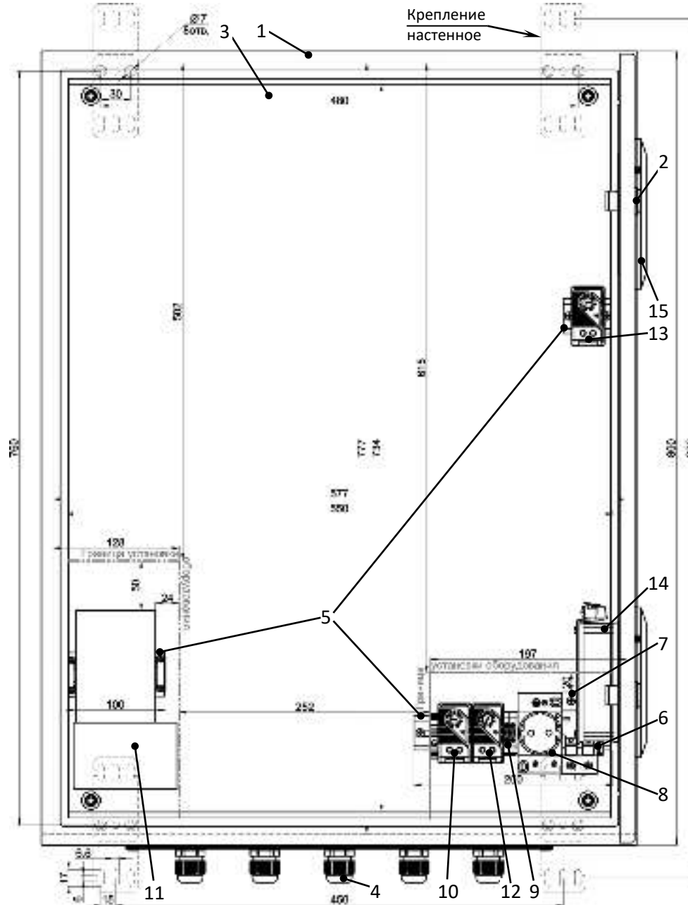
Рисунок 1 – Устройство шкафа
