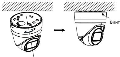
Рисунок 2-9 Установка камеры
