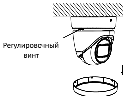
Рисунок 2-2 Регулировочные винты
