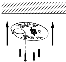
Рисунок 2-6 Крепление монтажной платформы
