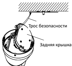
Рисунок 2-7 Крепление камеры к монтажной платформе
