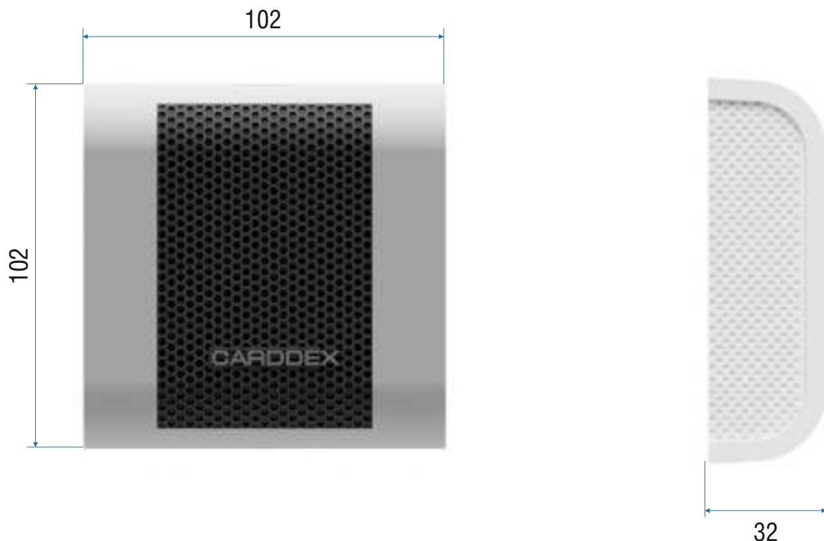
Рисунок 2.1 Габаритные размеры конвертера интерфейсов Ethernet/3RS-485 «CV E»
