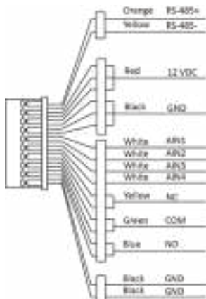
Рисунок 2-1 — Разъемы CTV-IP-D6000
