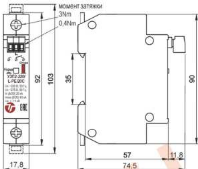
Рис.1 Габаритные размеры
