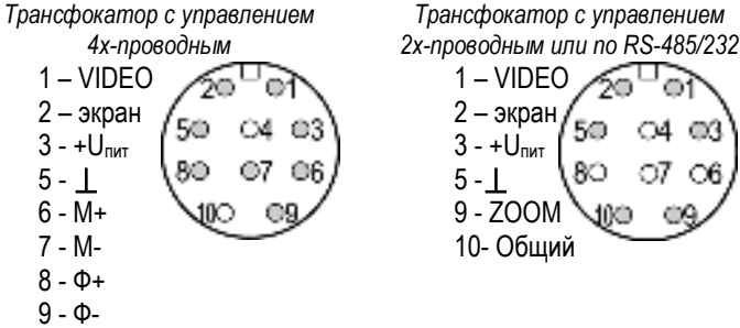
Рис.2 Распайка розетки РС-10 для объектива с трансфокатором (вид со стороны распайки проводников)
