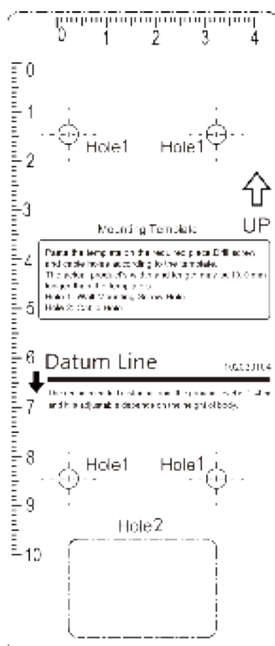
Рисунок 3-4 Монтажный шаблон
