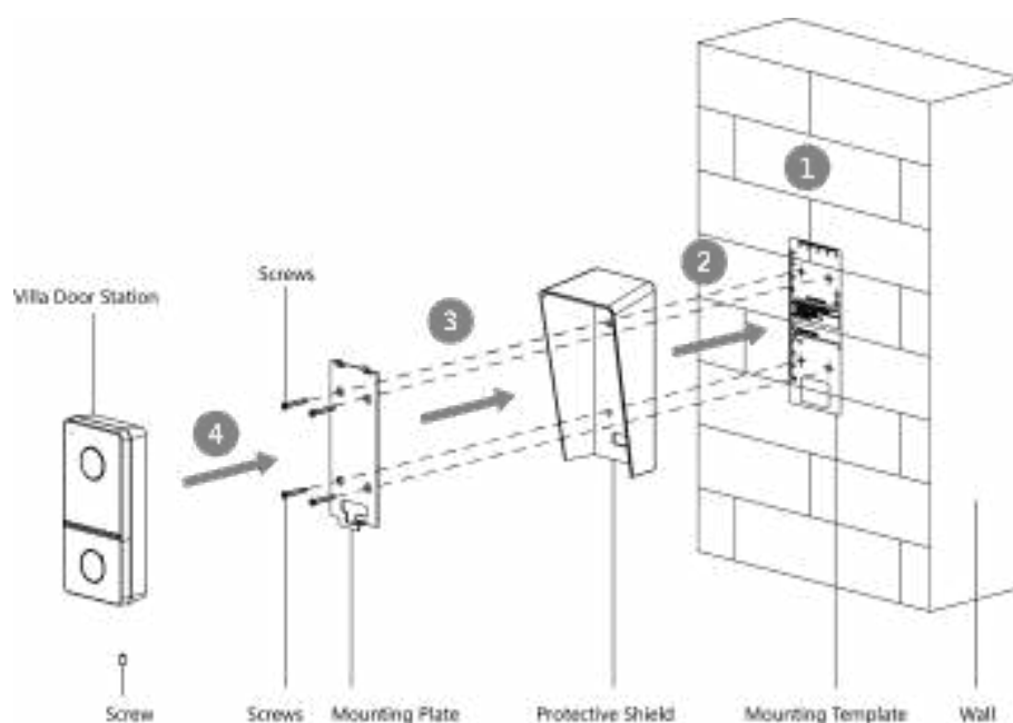
Рисунок 3-5 Накладная установка с защитным козырьком
