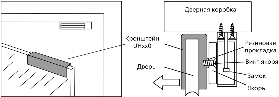
Рис.1 Монтаж на стеклянную дверь с помощью кронштейна U типа (UHxx0).
