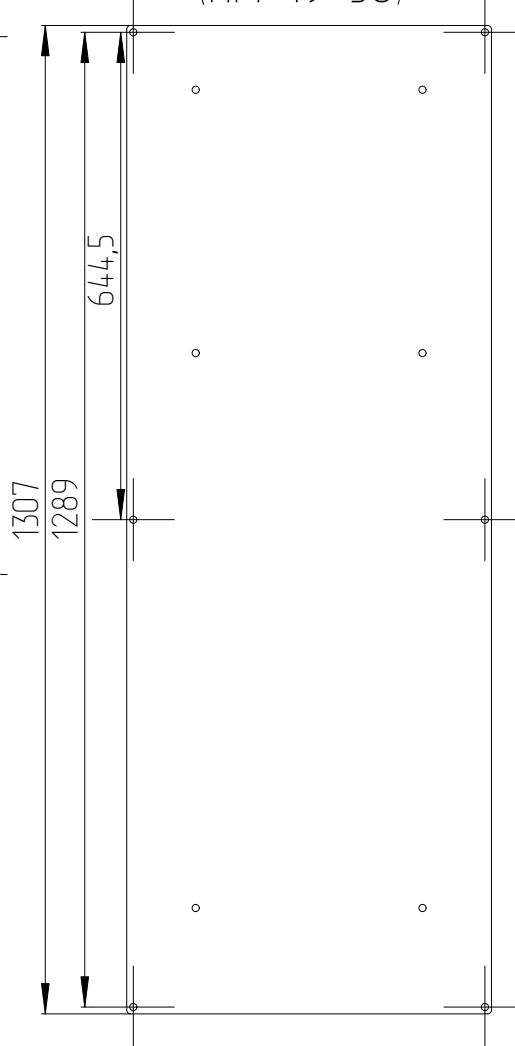
Панель ПМ-19"-30U (ПМ-19-30)
