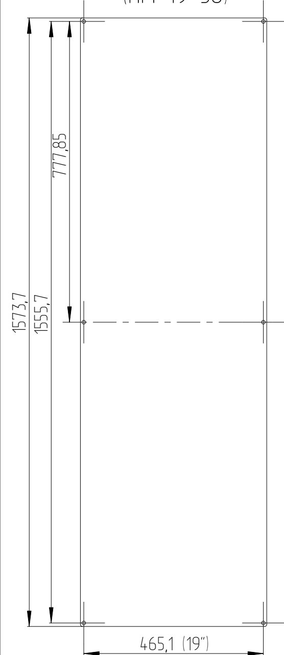
Панель ПМ-19"-36U (ПМ-19-36)
