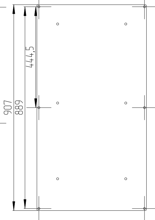
Панель ПМ-19"-21U (ПМ-19-21)
