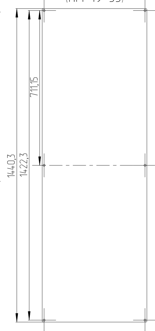
Панель ПМ-19"-33U (ПМ-19-33)
