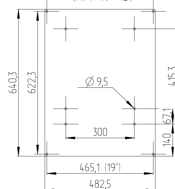
Панель ПМ-19"-15U (ПМ-19-15)
