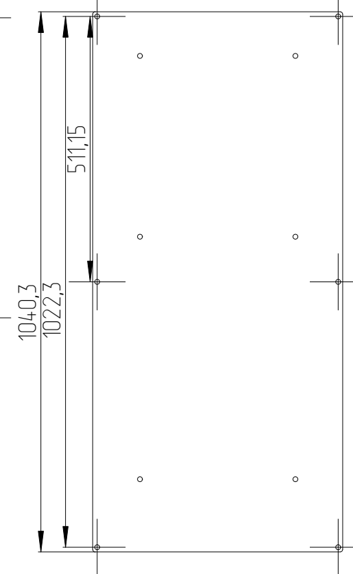
Панель ПМ-19"-24U (ПМ-19-24)
