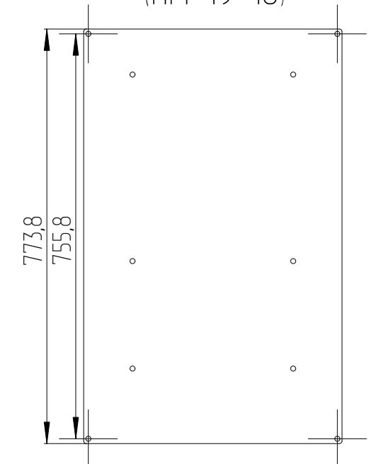
Панель ПМ-19"-18U (ПМ-19-18)
