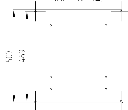
Панель ПМ-19"-12U (ПМ-19-12)
