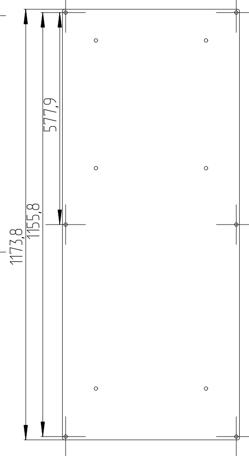
Панель ПМ-19"-27U (ПМ-19-27)
