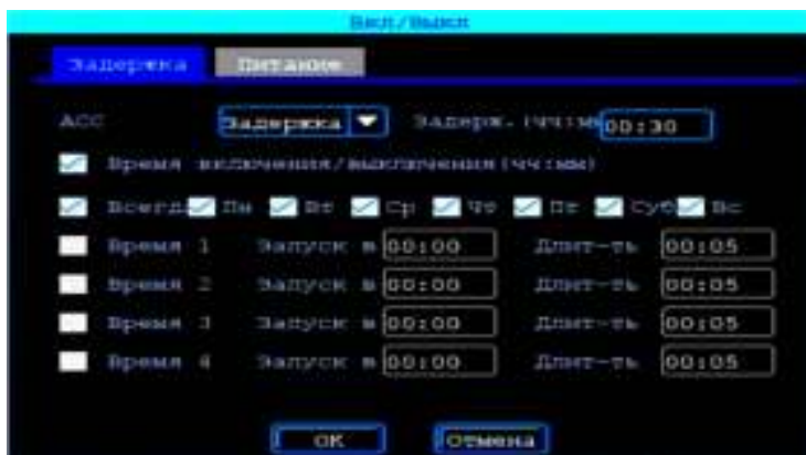
Рис.18 Настройки включения/выключения
