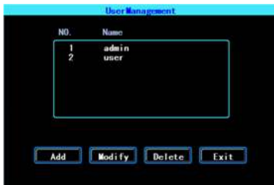
Рис.31 Управление пользователями
