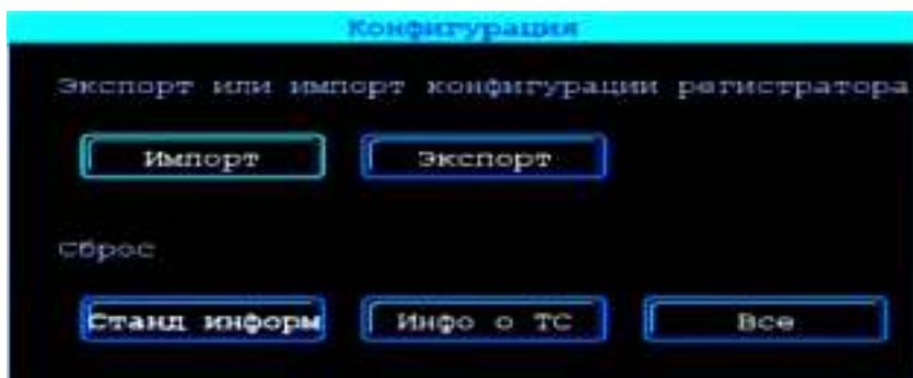
Рис.37 Импорт/Экспорт
