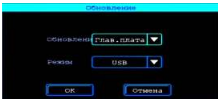
Рис.38 Обновление системы
