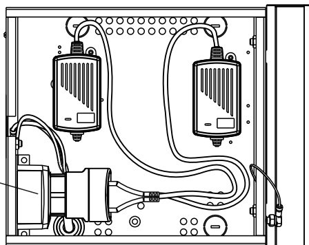
Рисунок 11 - Расположение двух блоков питания 19w/14.4v/EU FARADAY в боксе
