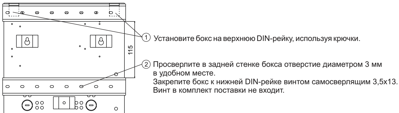
Рисунок 3 - Установка бокса на DIN-рейки
