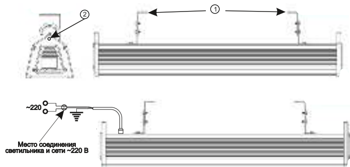
Рисунок 2 — Схема подключения изделия
