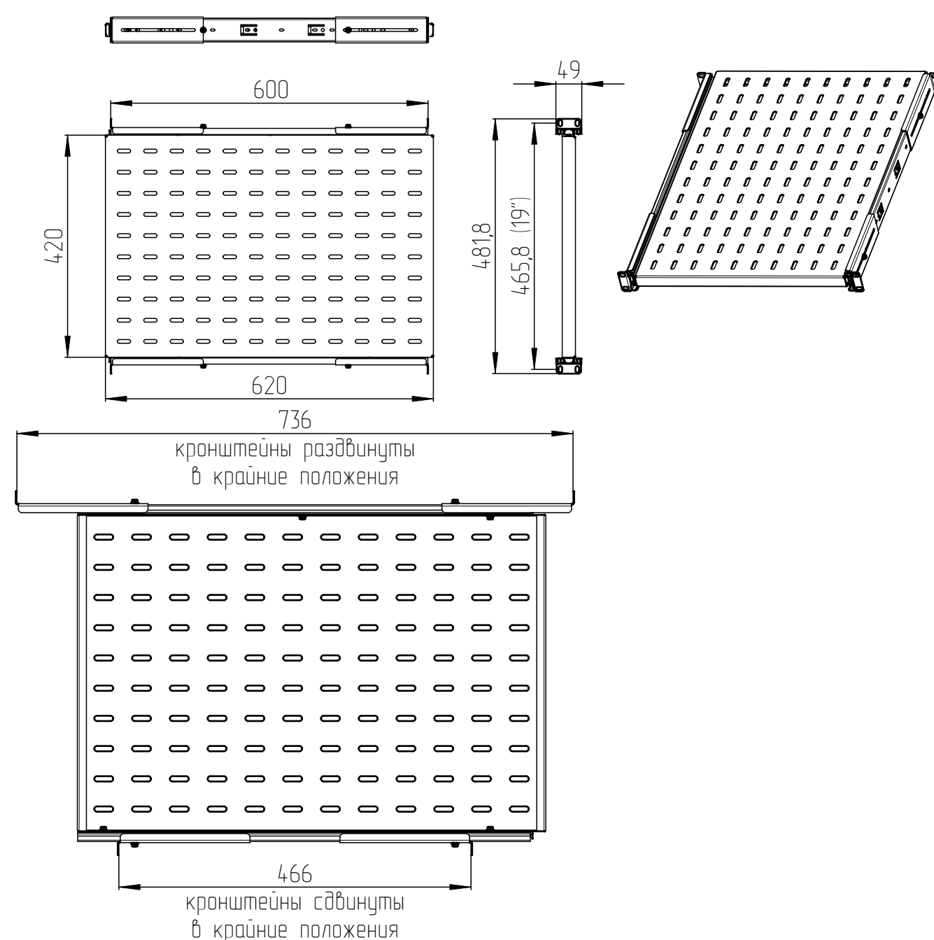
Полка ТСВ-КС
