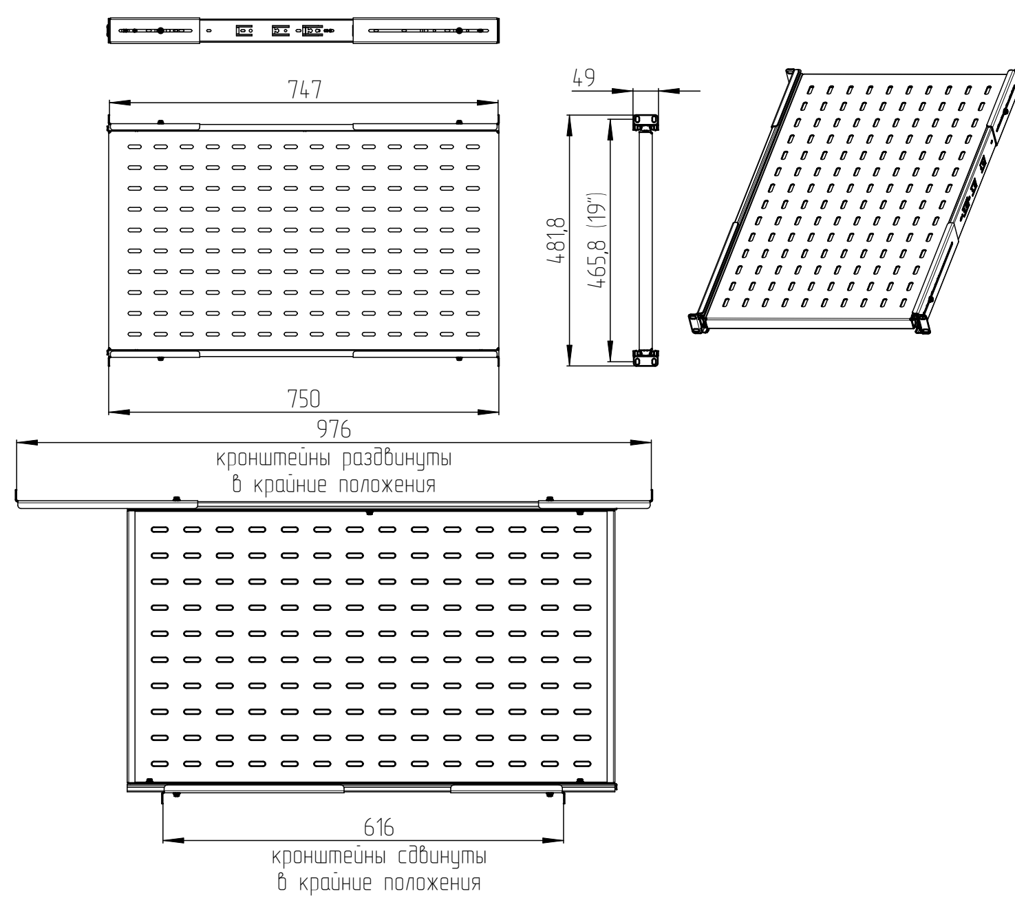
Полка ТСВ-К4
