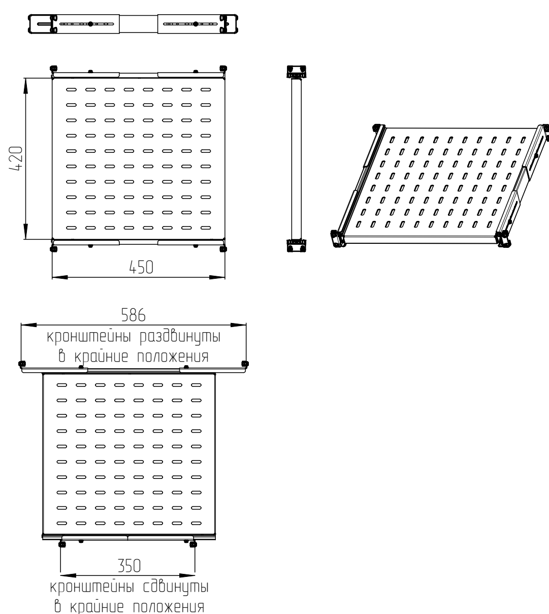
Полка ТСВ-45
