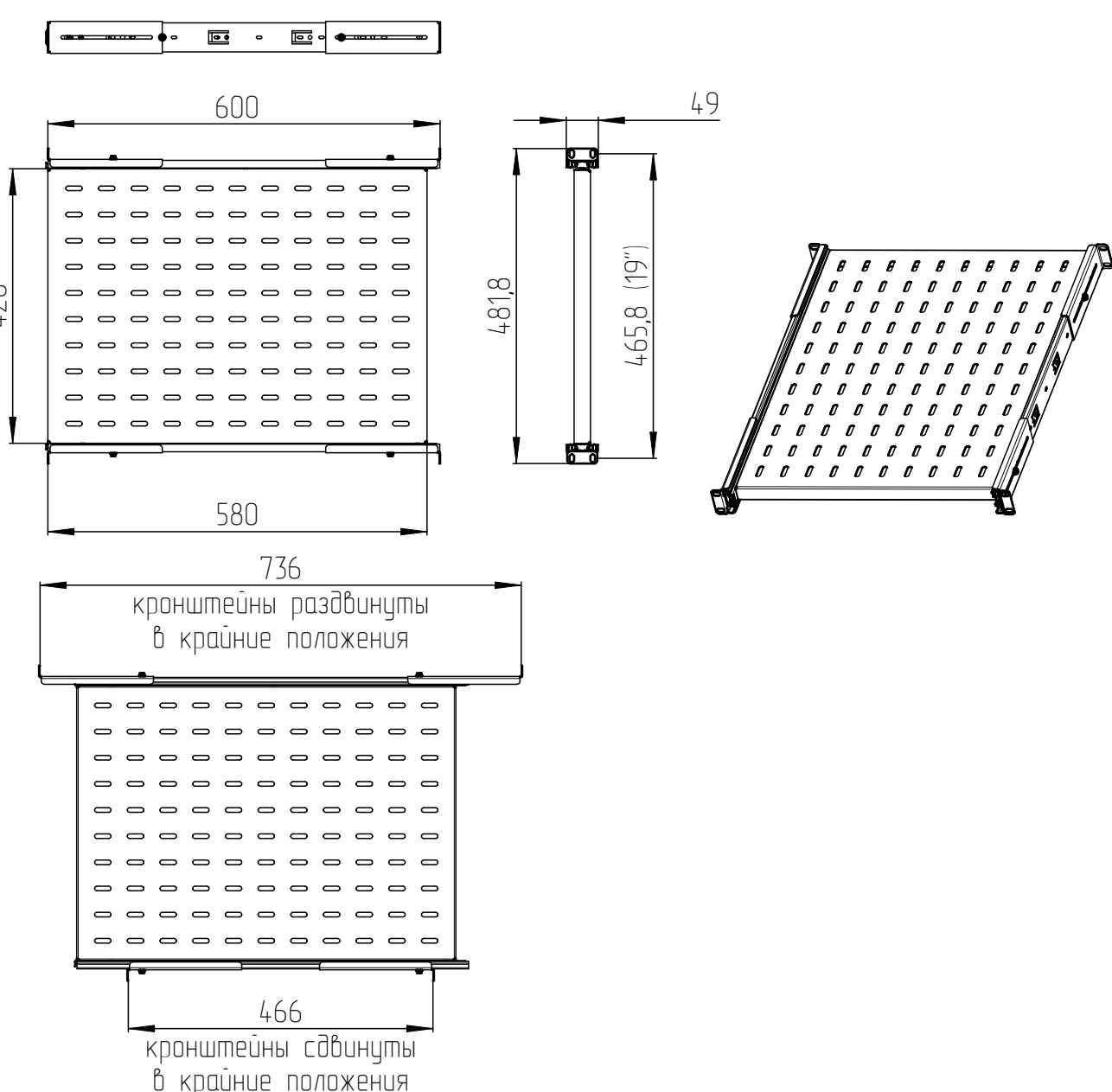
Полка ТСВ-45
