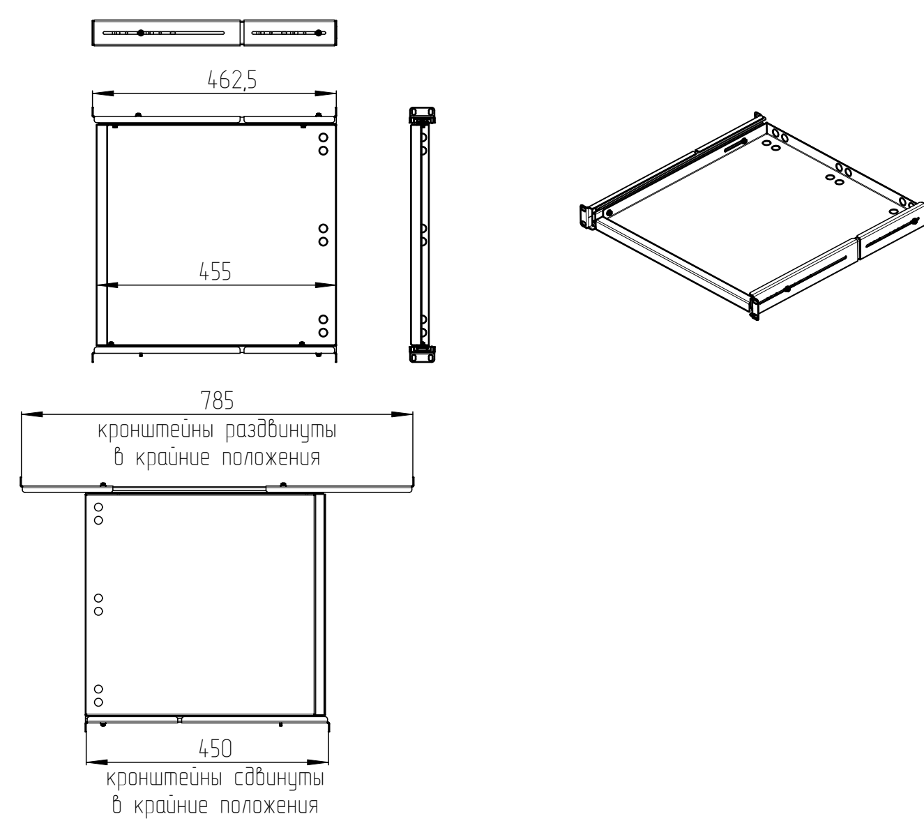
Полка ТСВ-К4
