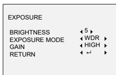
Рисунок 3-3 Меню EXPOSURE
