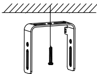
Рисунок 2-3 Установка кронштейна
