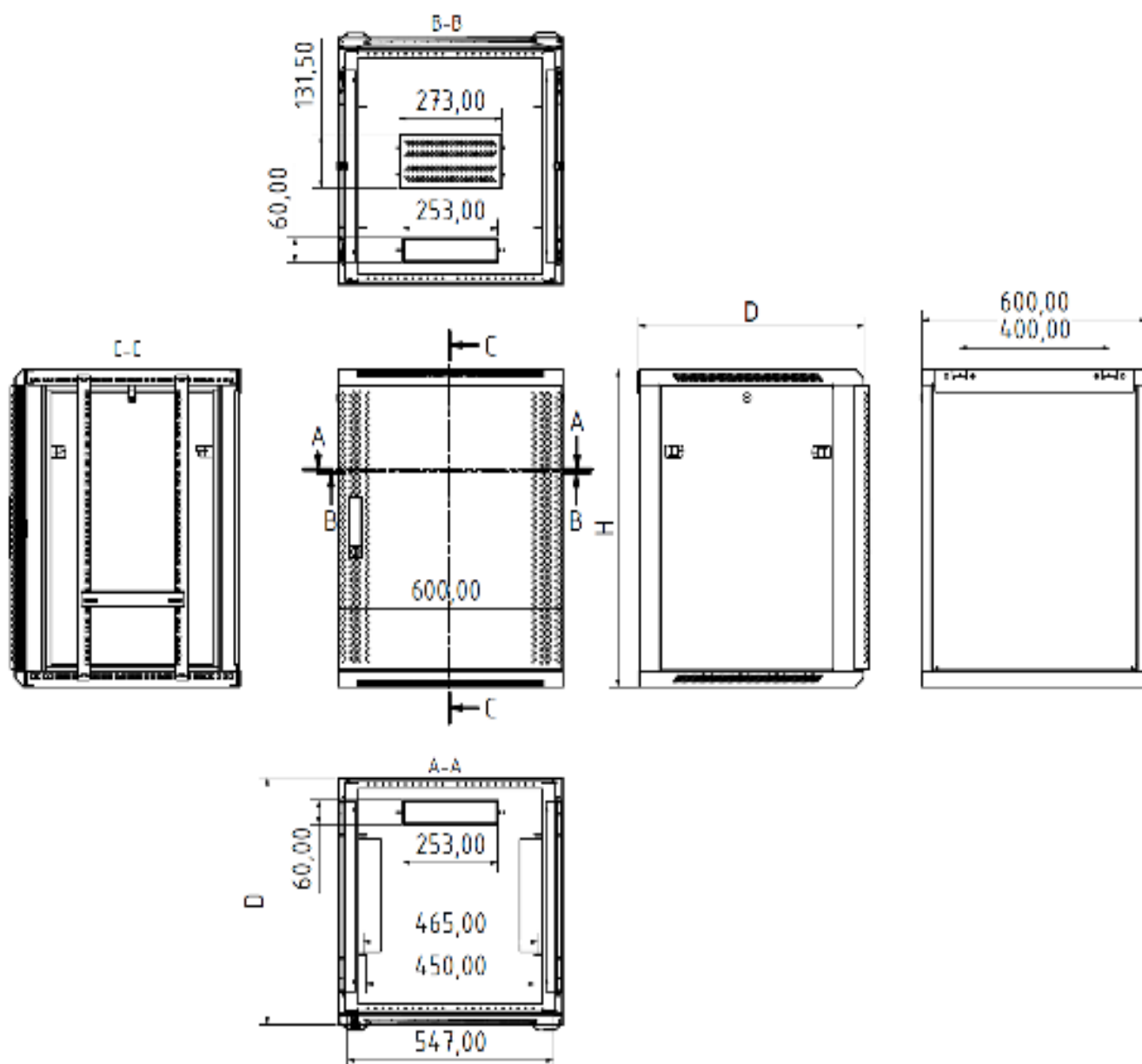
ЧЕРТЕЖ ШКАФА
