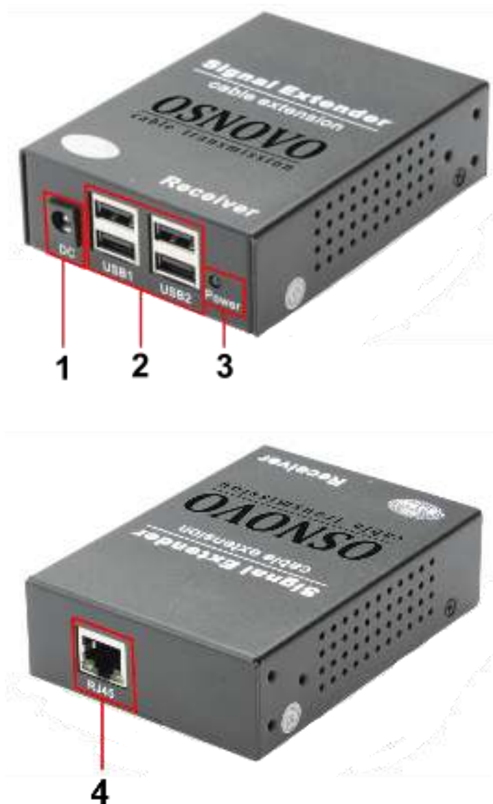
Рис. 4 Приемник RLN-U4/1, разъемы и индикаторы и задней панели
