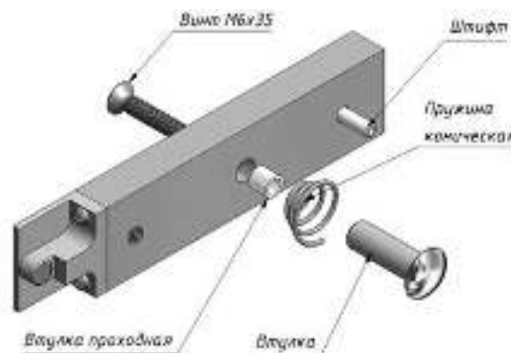
Рисунок 2 - Комплект крепления якоря
