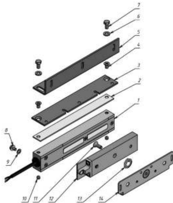
Рисунок 1 – Комплект поставки
