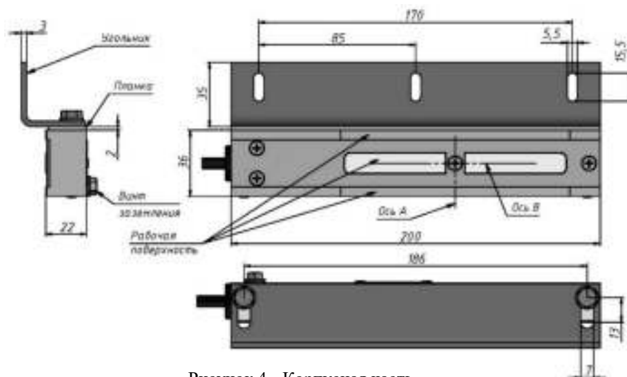
Рисунок 4 - Корпусная часть
