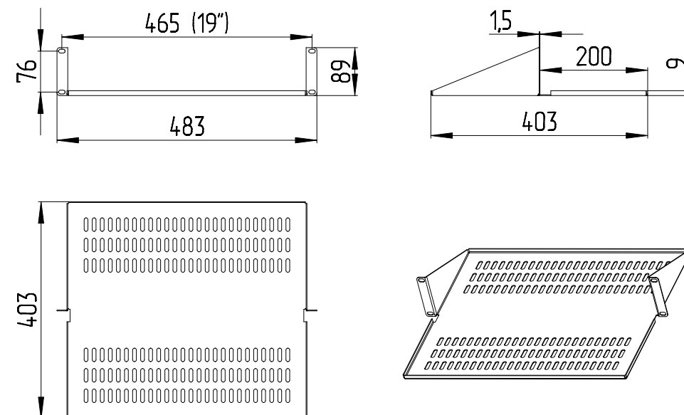
Полка МС-40.2
