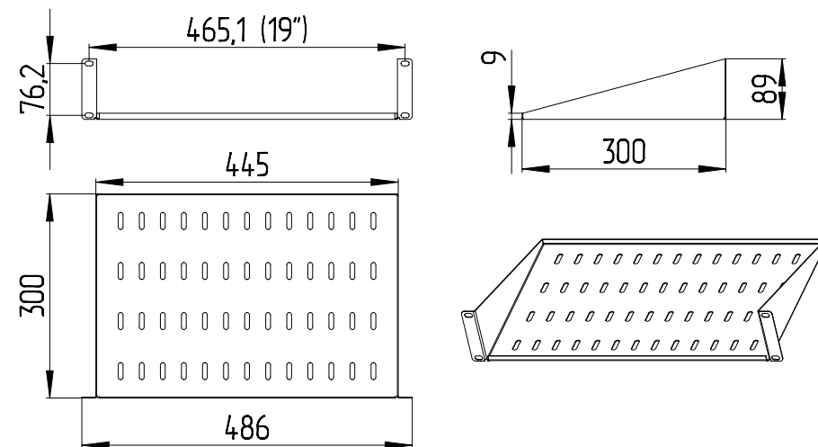
Полка МС-30
