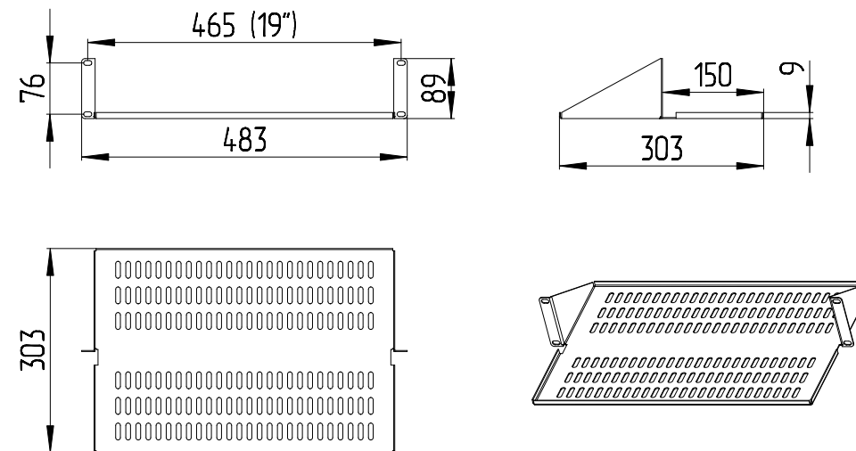
Полка МС-30.2
