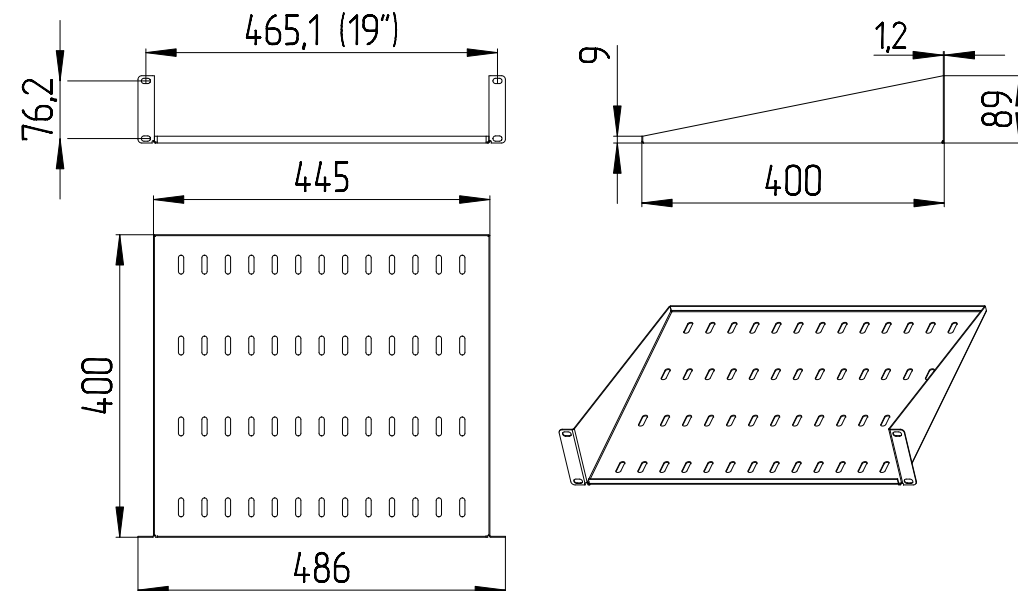
Полка МС-40
