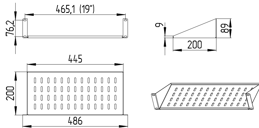
Полка МС-20
