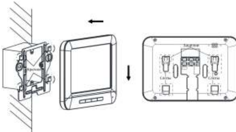
Рисунок 4-3 Установка видеодомофона на монтажное основание
