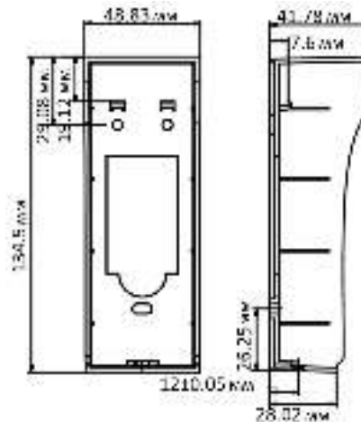
Рисунок 4-4 Монтажное основание
