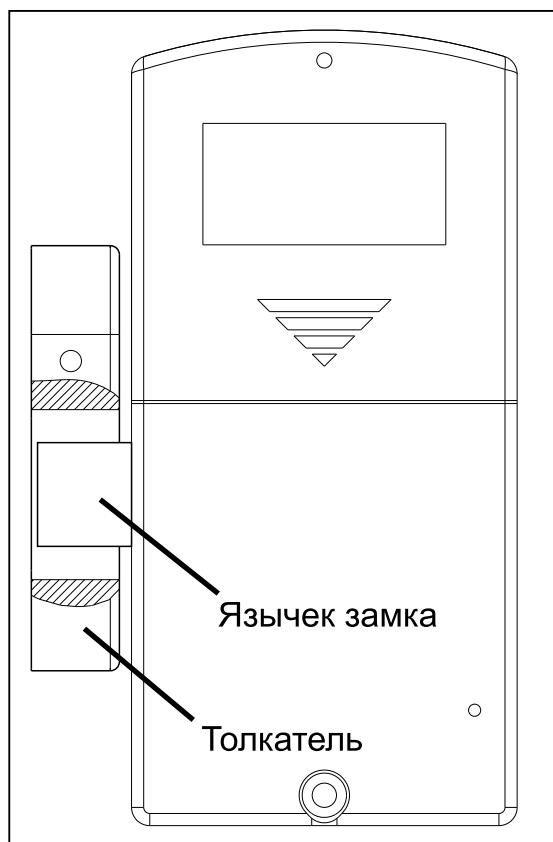
Рис. 7 Правильная установка. Вид с внутренней стороны двери
