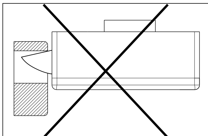
Рис. 6 Неправильная установка. Вид сверху
