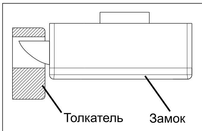
Рис. 5 Правильная установка. Вид сверху
