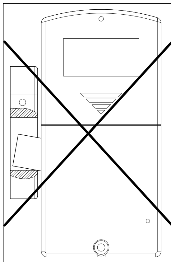
Рис. 8 Неправильная установка. Вид с внутренней стороны двери
